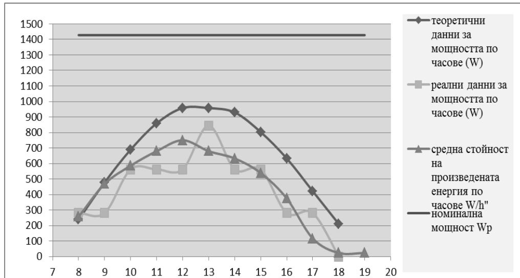
Фиг. 2. Изменение на мощността на фотоволтаичната система по часове.
