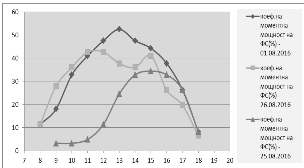
Фиг. 3. Изменение на коефициента на мощност.
